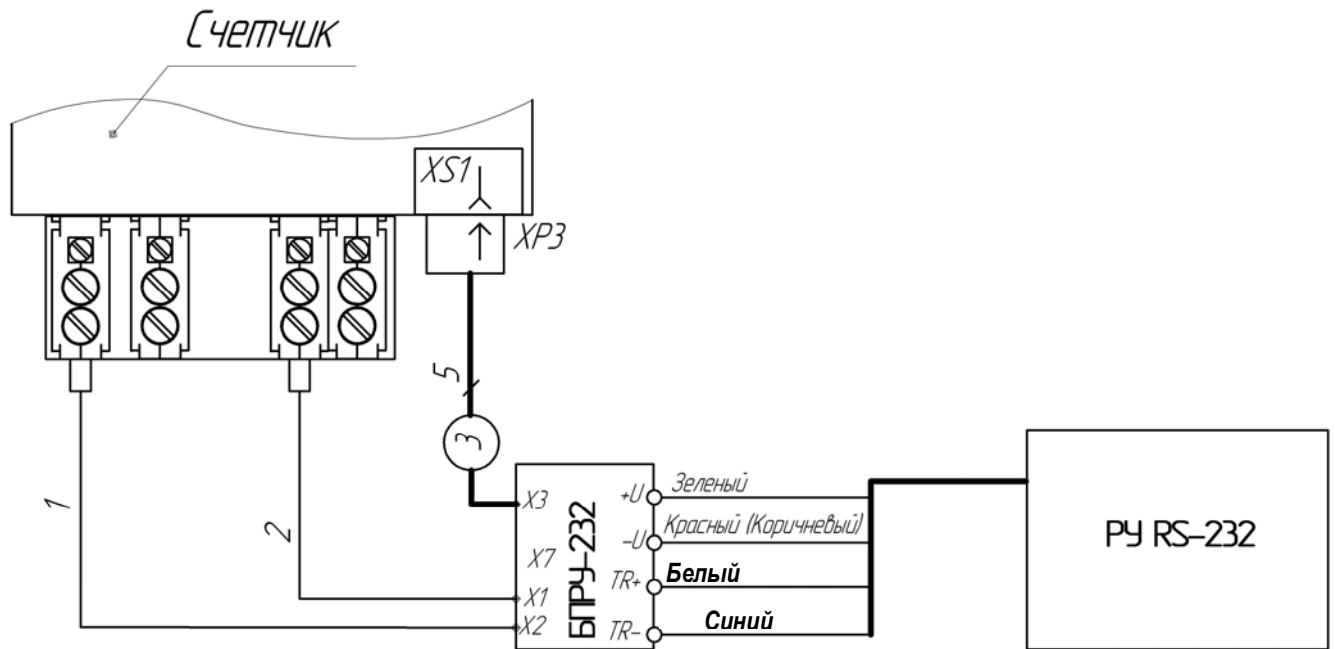
Рисунок 1 — Схема подключения УРК РМ062.01
