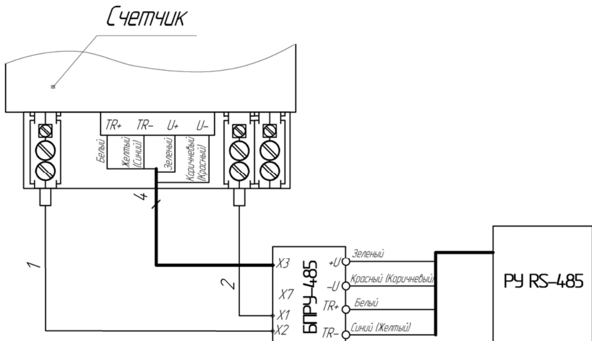
Рисунок 2 — Схема подключения УРК РМ012.01
