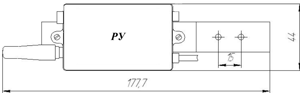
Рисунок А.2 — Габаритные и установочные размеры радиоудлинителя RS-232 (RS-485)
