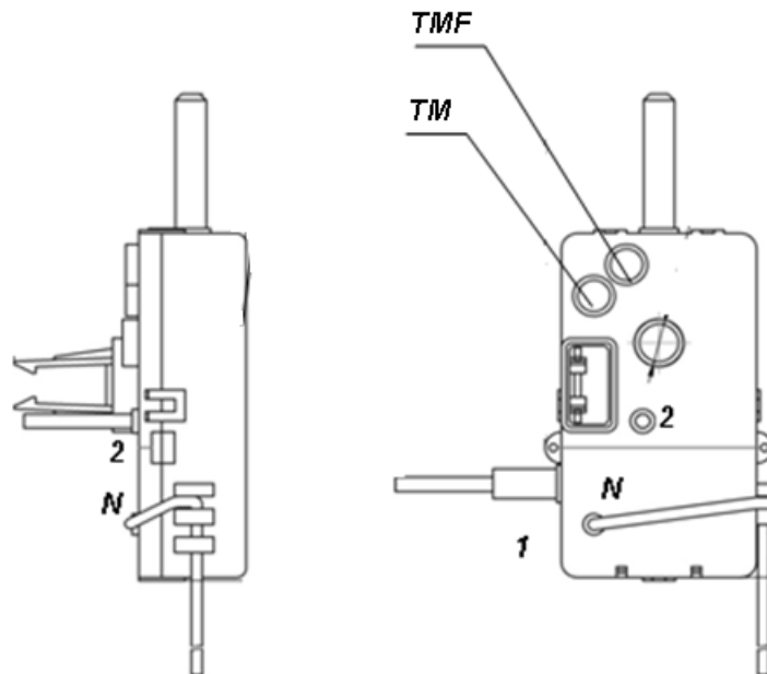
Рисунок Г.2 – Схема расположения контактов и индикаторов счетчиков РиМ 129.02, РиМ 129.04
