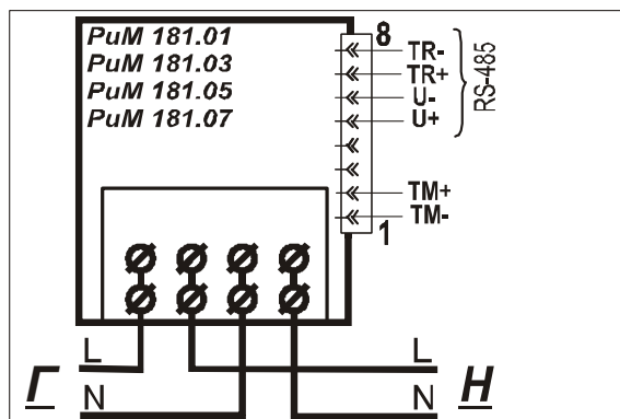
Рисунок 1 – Схема подключения счетчиков РИМ 181.01, РИМ 181.03, РИМ 181.05, РИМ 181.07
