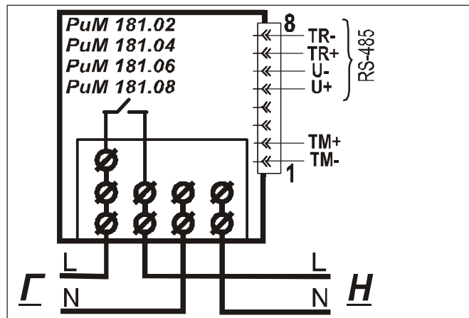
Рисунок 2 – Схема подключения счетчиков РИМ 181.02, РИМ 181.04, РИМ 181.06, РИМ 181.08
