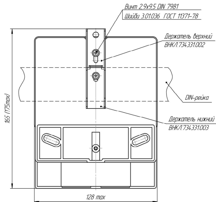
Рисунок 3 – Схема установки счетчиков на DIN-рейку
