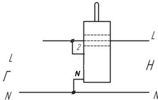
Рисунок 2 – Схема подключения счетчиков РИМ 189.11, РИМ 189.13
