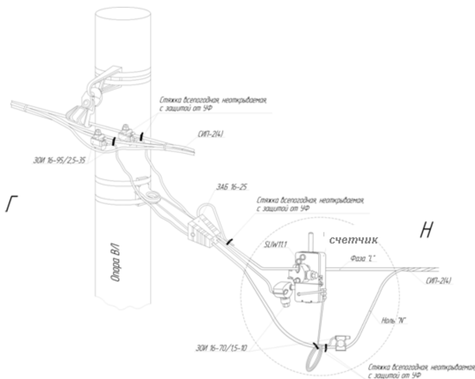
Рисунок 3 - Схема подключения счетчика
