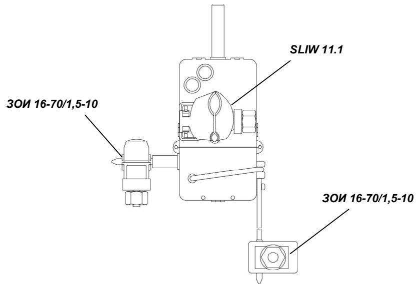
Рисунок 1 - Габаритные, установочные размеры и расположение индикаторов счетчиков
