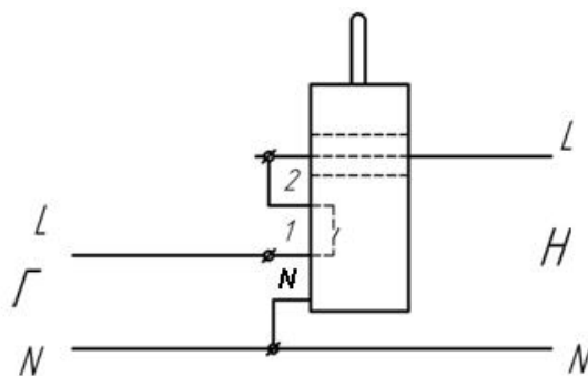
Рисунок 3 - Схема подключения счетчика
