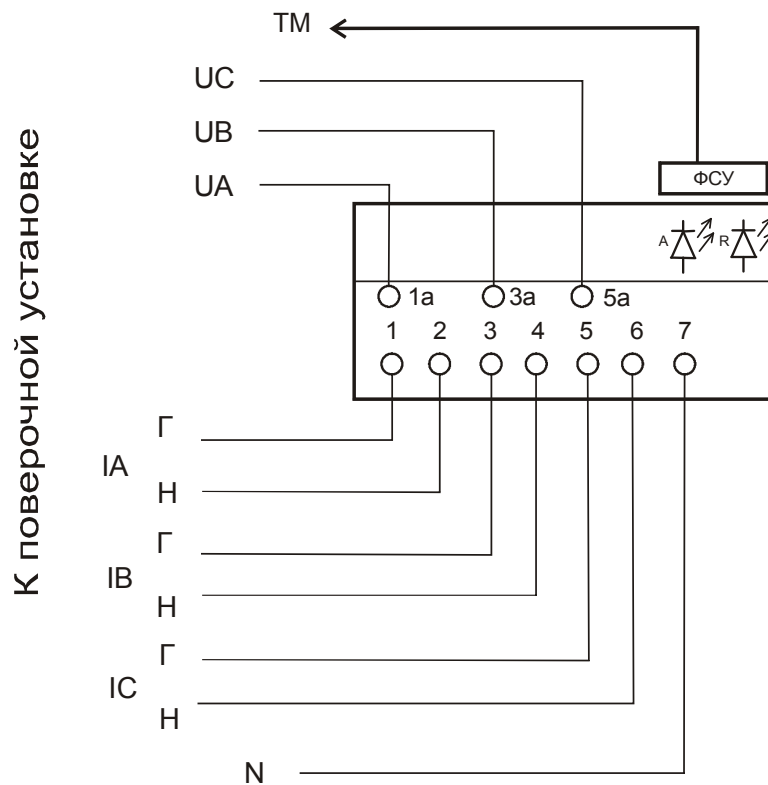
Рисунок Б.3 – Схема включения счетчиков в корпусе типа 2 (контакты 1а, 3а, 5а доступны, см. рисунок Г.2) при проведении опробования, проверке работоспособности оптического испытательного выхода, допускаемой основной погрешности, вызываемой изменением тока, дополнительной погрешности, вызываемой изменением напряжения в установленном диапазоне
