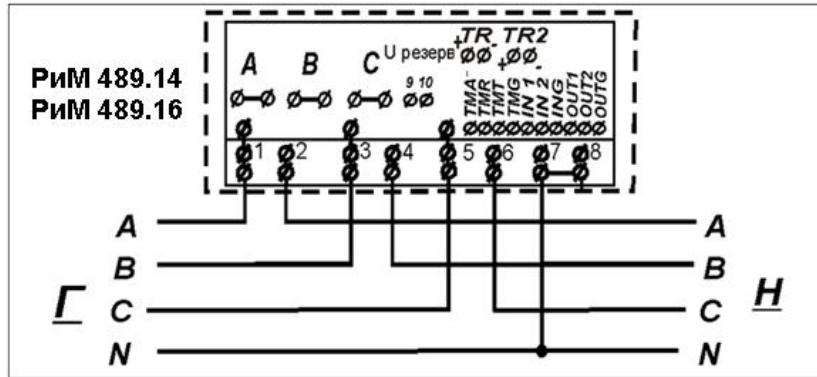
Рисунок 1 – Схема подключения счетчиков
